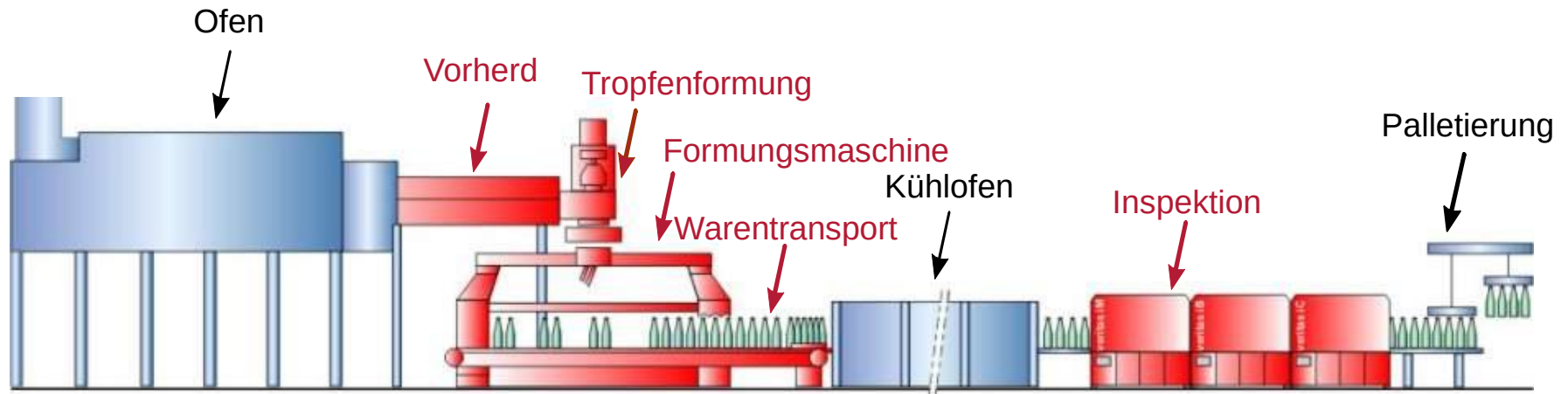
Glasbehälterverarbeitungsprozess
