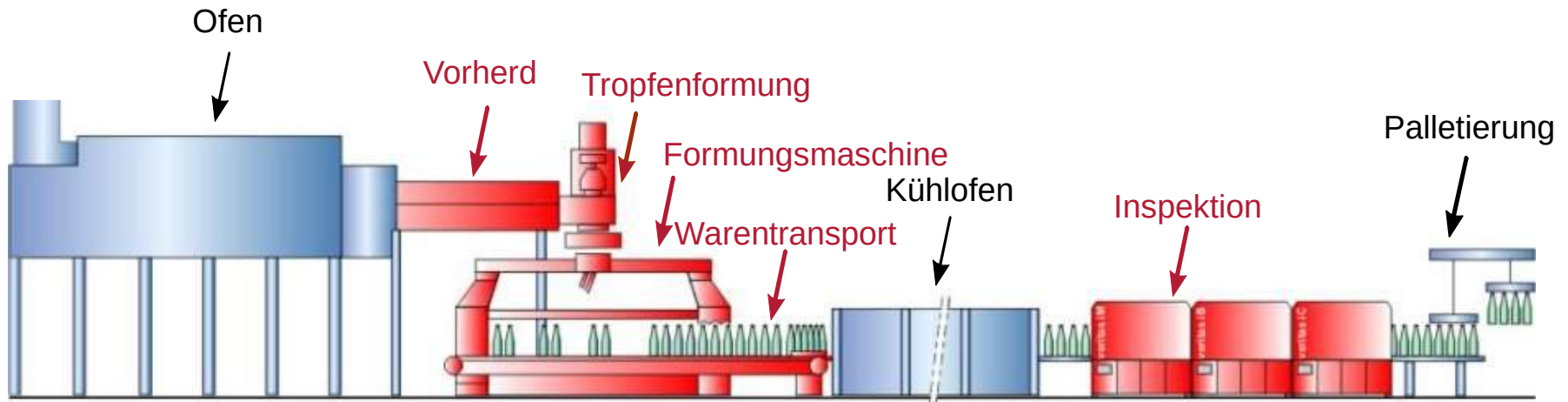
Glasbehälterverarbeitungsprozess
