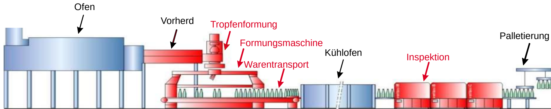
Glasbehälterverarbeitungsprozess
